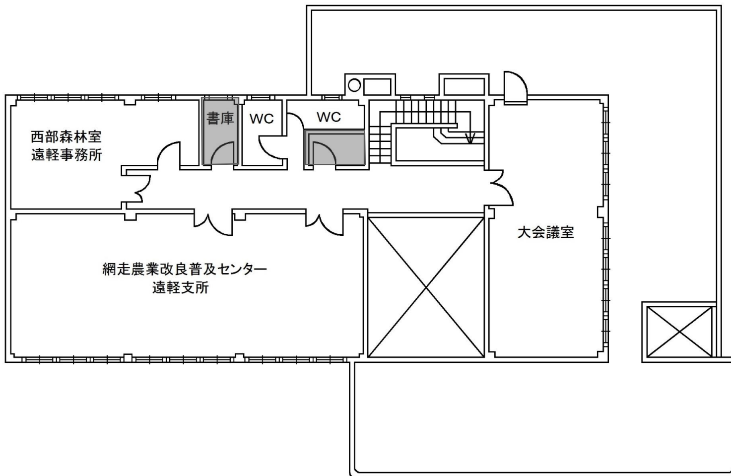
遠軽合同庁舎2階平面図
